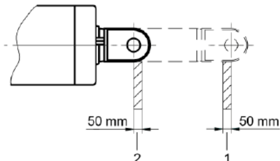
Rysunek 30 Dopuszczalna redukcja skoku silnika Picoło
