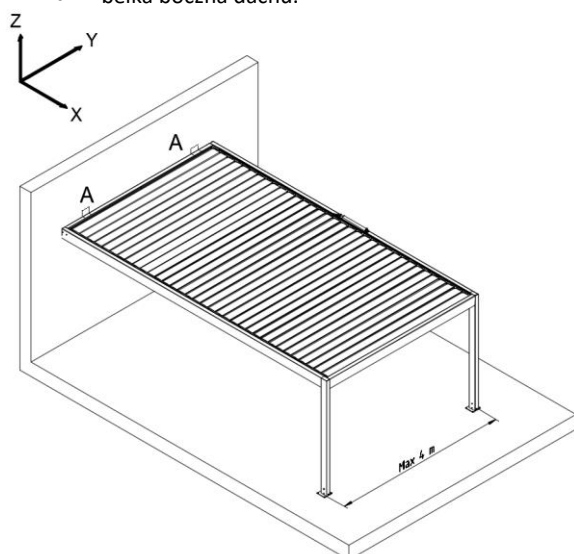
A – Uchwyty ścienny montowane do węzła belek.
