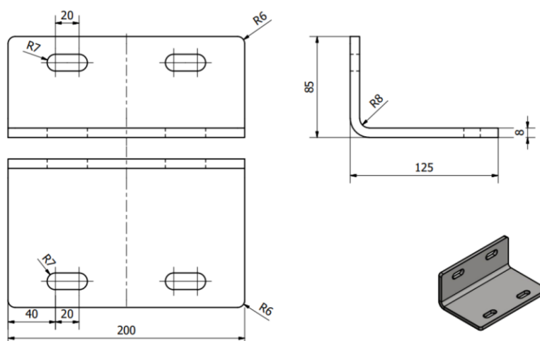
Rysunek 33A – Uchwyt przyścienny uniwersalny – wersja gięta (zastępuje obie wersje gorącowalcowane).
