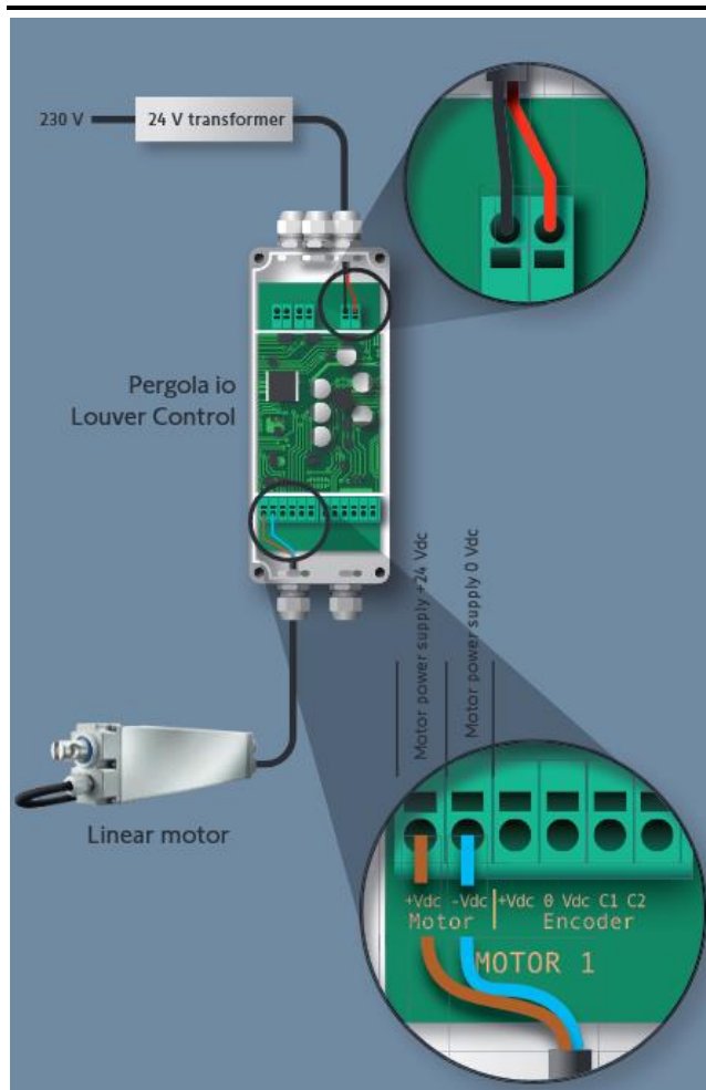
Rys. 36 Schemat obszarów podłączeń wewnątrz centralki Pergola io Louver (opisy na dolnym powiększeniu podano jako pogrubione w tabeli powyżej)
