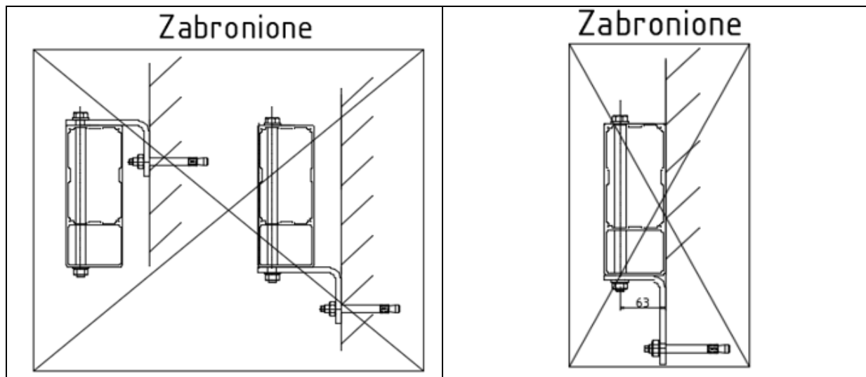
Rysunek 33B – Uchwyt przyścienny uniwersalny – zabronione sposoby mocowania.
