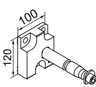
Uchwyty ścienny prawa
