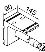
Konsola stropowa prawa
