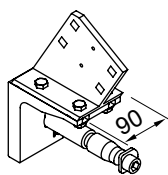
Wspornik krokwiowy nakładka: 150 mm prawa
