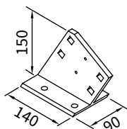
Wspornik krokwiowy 90 mm wysokość płaskownika 150 mm
