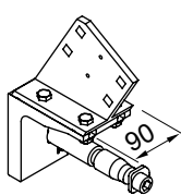
Wspornik krokwiowy nakładka: 150 mm
