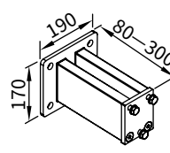
Wspornik dystansowy 80–300 mm do uchwyty ściennego 100 mm z separatorem termicznym
