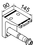
Konsola stropowa lewa
