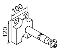
Uchwyt ścienny prawa
