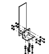
Nakładka i kątownik do mocowania do krokwi nakładka: 500 mm
