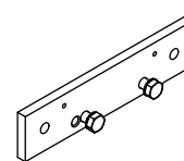
Dodatkowa nakładka krokwi do konsoli krokwiowej
