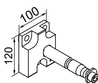
Uchwyt ścienny prawa
