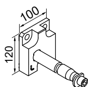
Uchwyty ścienny lewa
