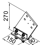
Wspornik krokwiowy 90 mm wysokość płaskownika 270 mm
