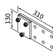
Płyta mocująca C 310 × 130 × 12 mm
