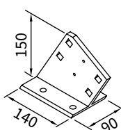
Wspornik krokwiowy 90 mm wysokość płaskownika 150 mm
