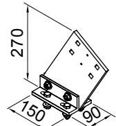
Wspornik krokwiowy 90 mm wysokość płaskownika 270 mm
