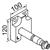
Uchwyt ścienny lewa
